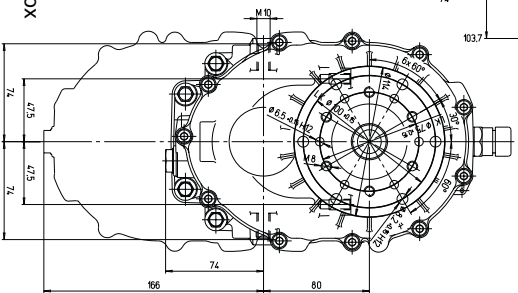
C-Getriebe C-type gearbox
