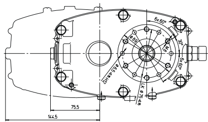
B-Getriebe B-type gearbox
