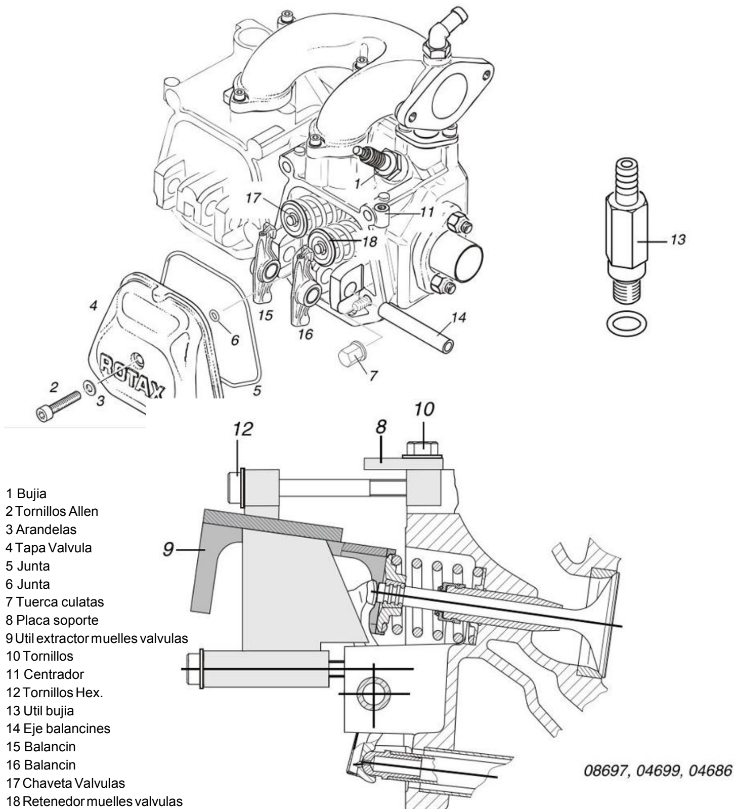
Fig.2 Tren de Valvulas
